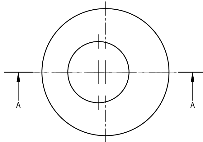
Casquillo aislante excentrico diam 26
